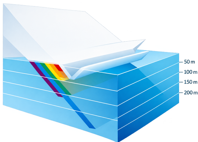
Figur 14: Lysabsorption i havet og tiltagende mørke i dybet [12].
