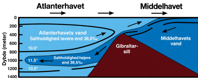
Figur 12: Middelhavsvand flyder ind i Atlanterhavet over Gibraltar-tærsken som en saltholdig, varm vandmasse, der bevarer sine fysiske egenskaber [21].
