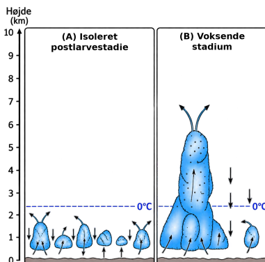
Figur 17: Skyerne smelter sammen og vokser lodret via indre opvinde [3].
