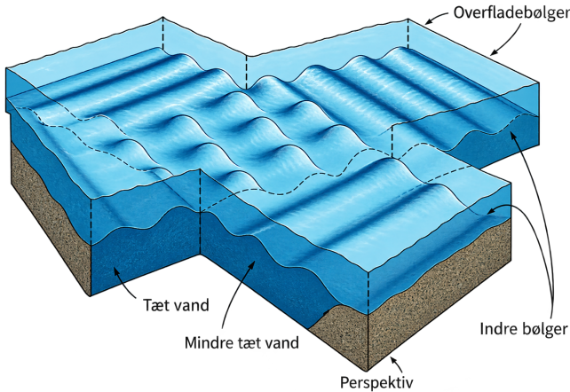
Figur 15: Interne bølger der udbreder sig langs tæthedsgrænsen mellem vandmasser under overfladen [16].
