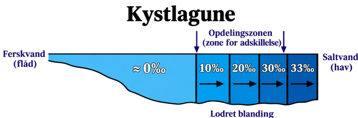
Figur 13: Længdesnit gennem en flodmunding der viser saltholdighedsgradienten og overgangszonen mellem ferskvand og saltvand [16].
