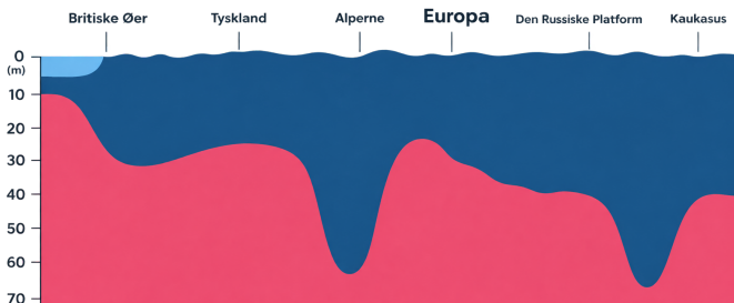
Figur 7: Skematisk geologisk tværsnit, der illustrerer bjergenes dybe rødder (isostasi) [39].
