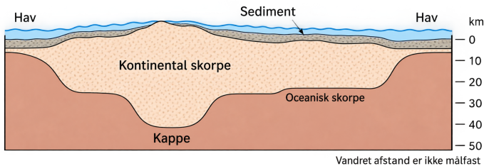
Figur 6: Bjerger har dybe underjordiske rødder indlejret i litosfæren, ganske som teltpløkker [33].
