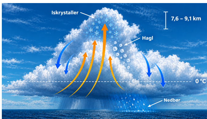
Figur 18: Cumulonimbusky der rager op som et bjerg i atmosfæren [3].
